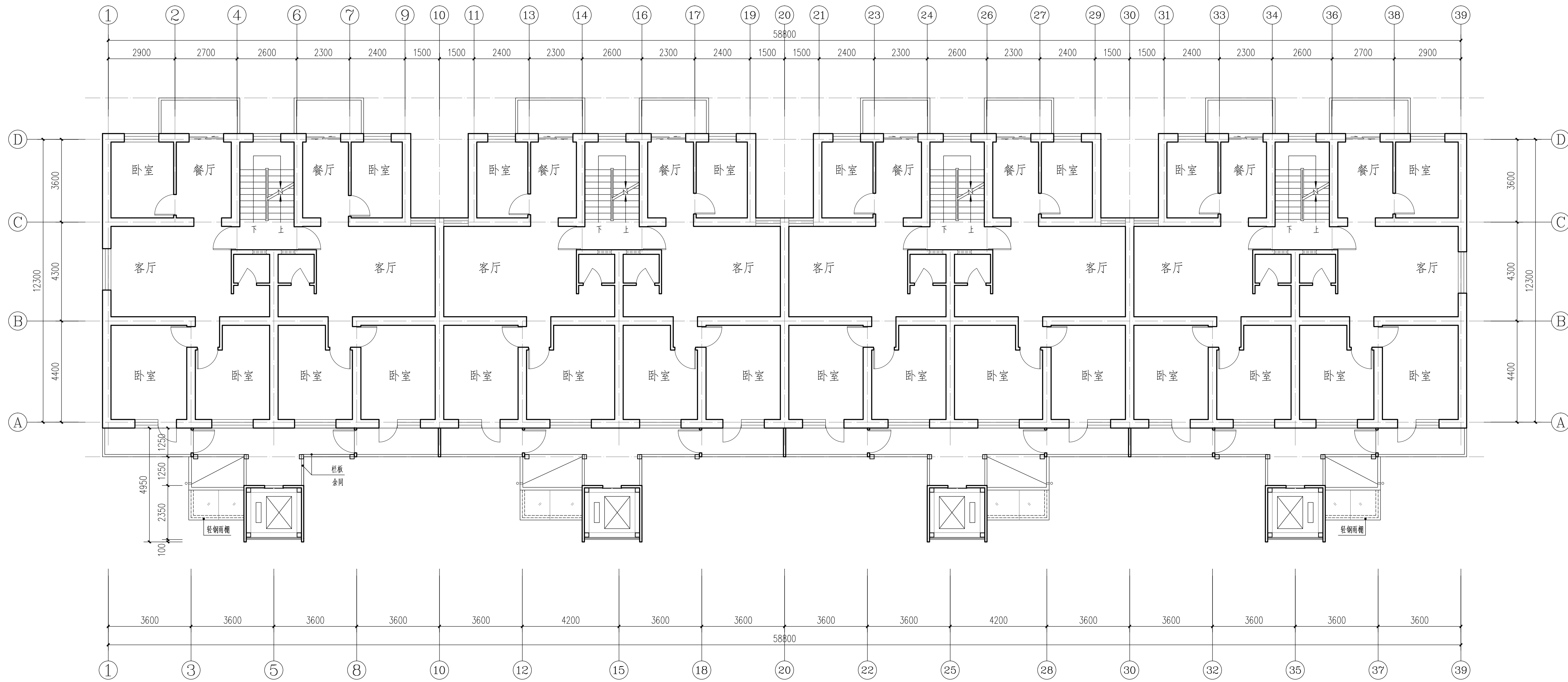
1#楼标准层平面 1:100
