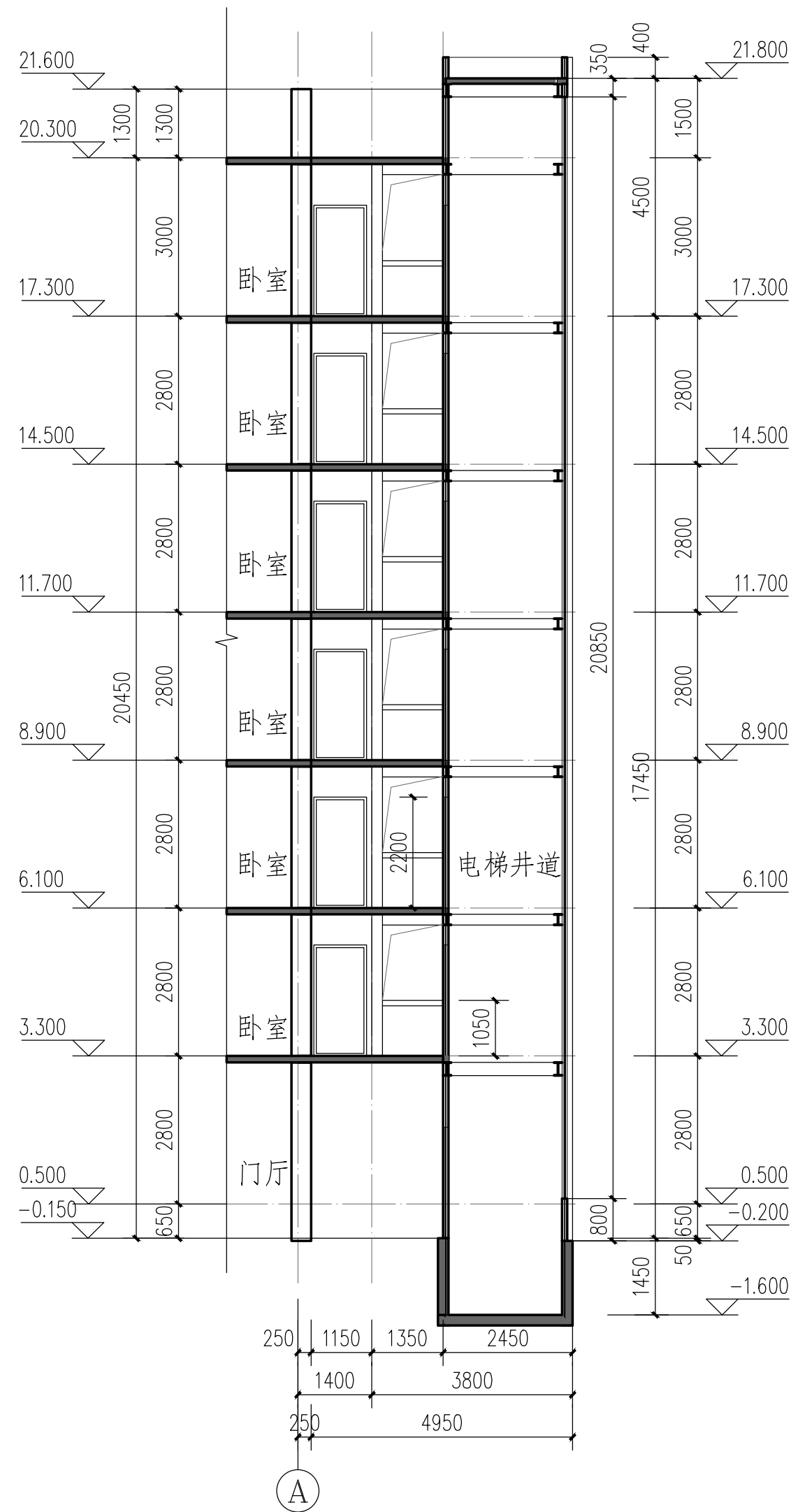
1-1剖面图 1:100
