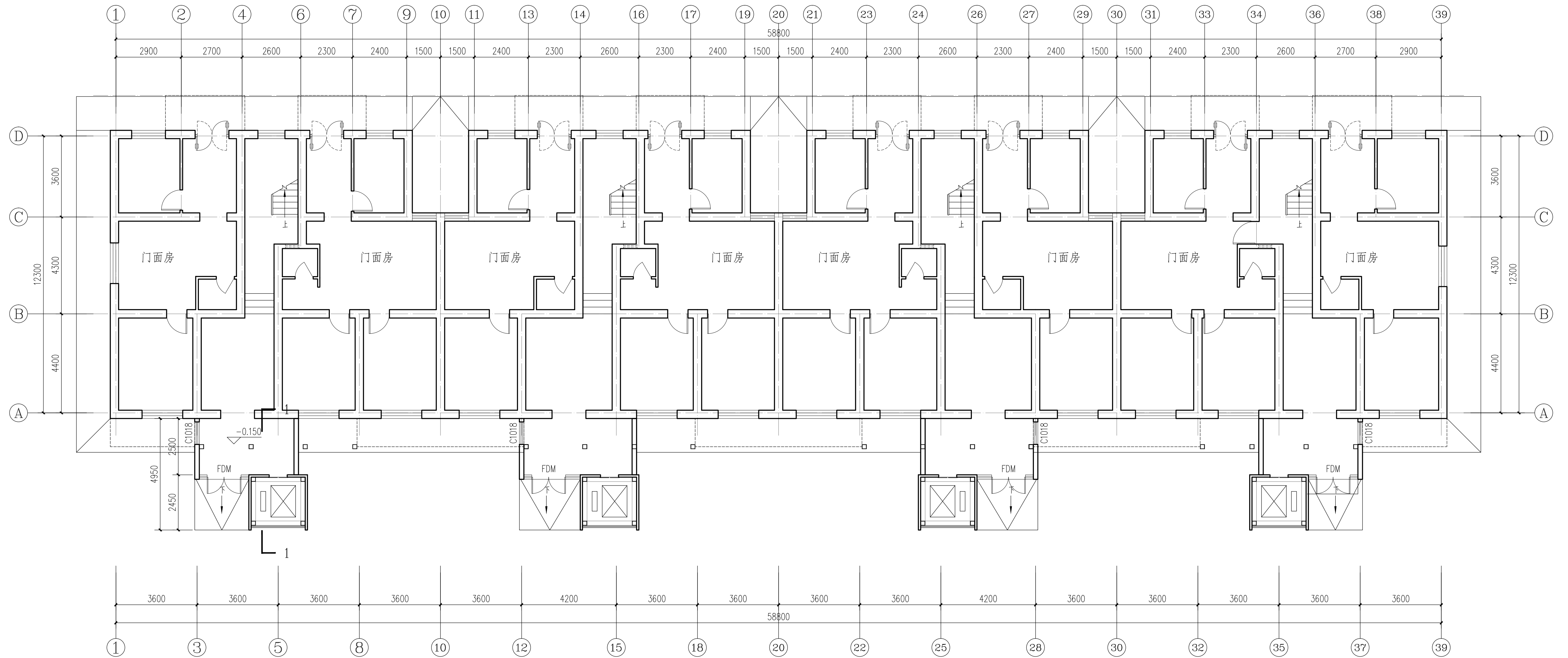
1#楼首层平面 1:100
