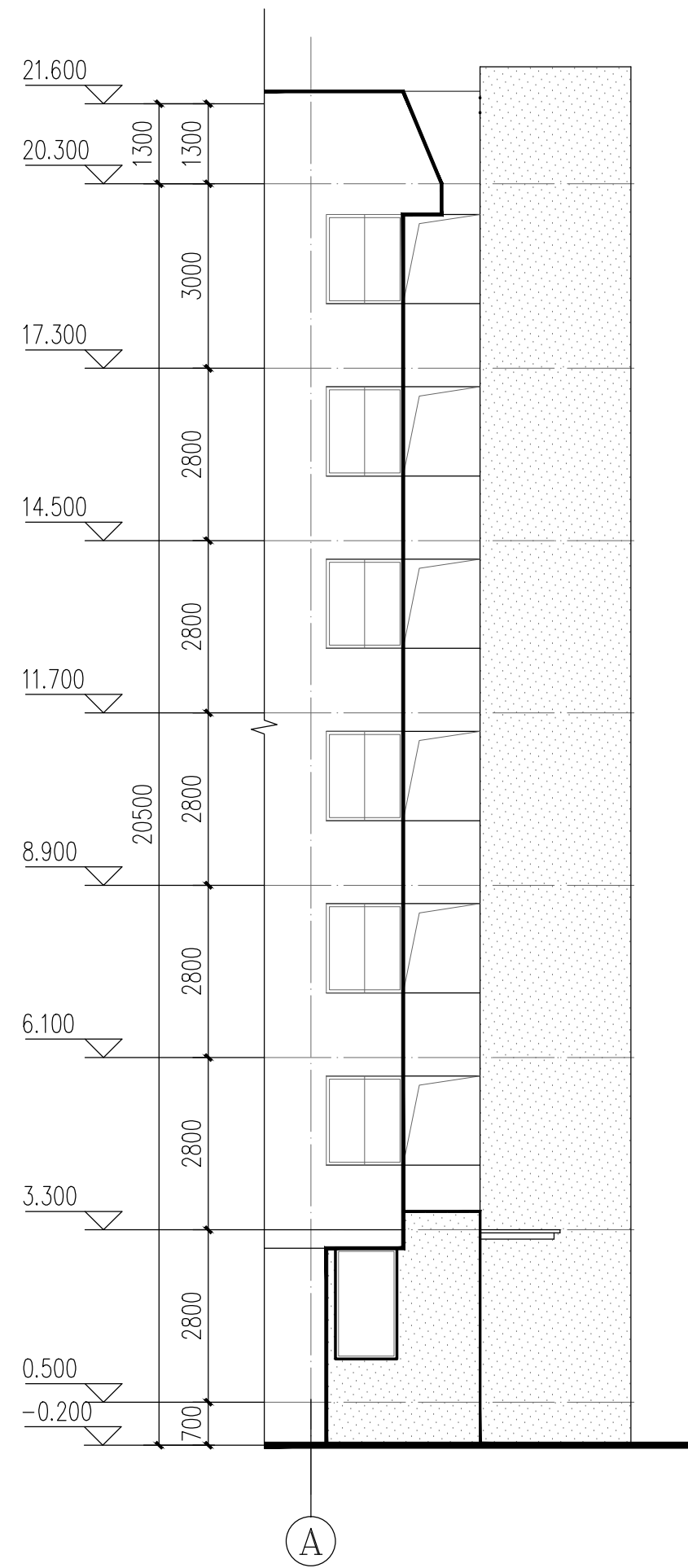
侧立面 1:100
