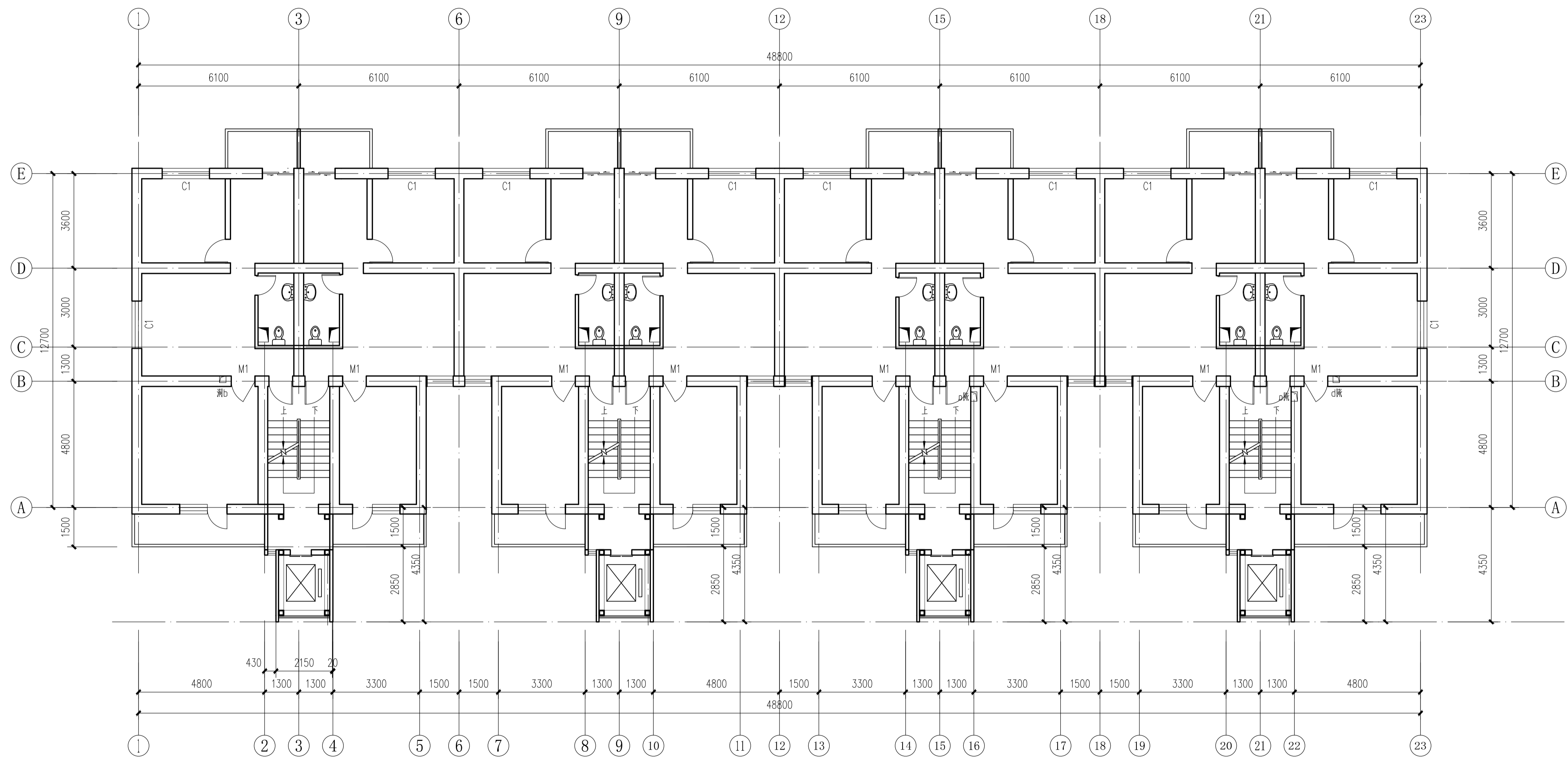
22#楼二-七层平面 1:100
